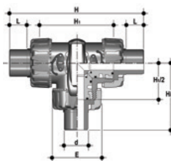
ТРЕХХОДОВОЙ ШАРОВОЙ КРАН DualBlock® с гладкими втулочными окончаниями, метрическая серия
