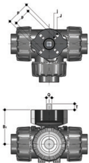
Модульный адаптор для пневмопривода
