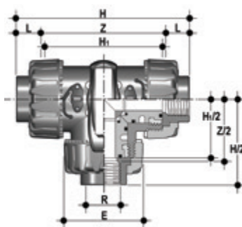
ТРЕХХОДОВОЙ ШАРОВОЙ КРАН DualBlock® с окончаниями с внутренней цилиндрической резьбой BS
