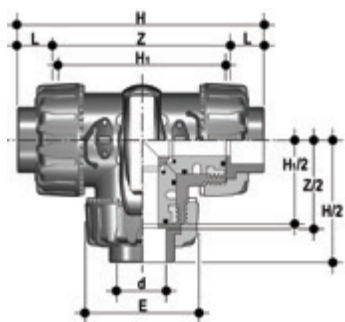
ТРЕХХОДОВОЙ ШАРОВОЙ КРАН DualBlock® с гладкими муфтовыми окончаниями, метрическая серия
